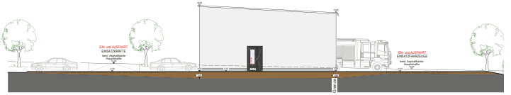
NORDWESTANSICHT
